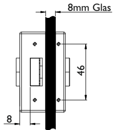
Bohrschema
