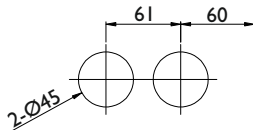
Bohrschema
